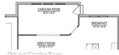
Optional Carolina Room
